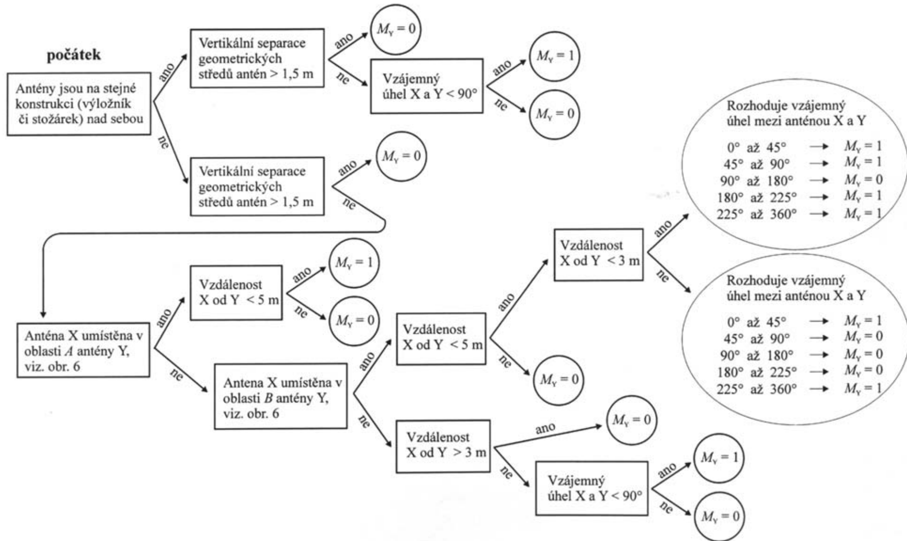
Obr. 4 Diagram, který každé dvojici antén X a Y přiřadí koeficient M_V
