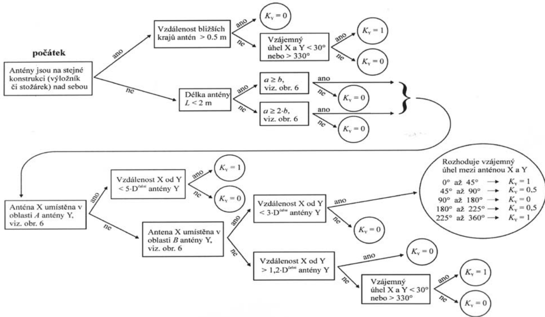
Obr. 5 Diagram, který každé dvojici antén X a Y přiřadí koeficient K_V
