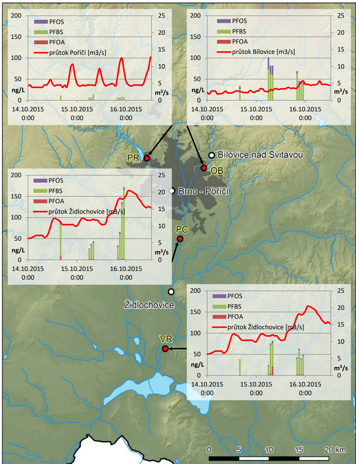
Mapa č. 33 Denní variabilita koncentrace perfluorovaných látek při různých průtocích ve vodních útvech v městské aglomeraci Brno.
